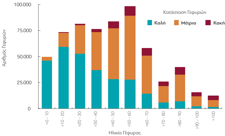
Πηγή: InfoBridge. Διαθέσιμο στο: https://infobridge.fhwa.dot.gov/Data/BridgeDetail/20656192
